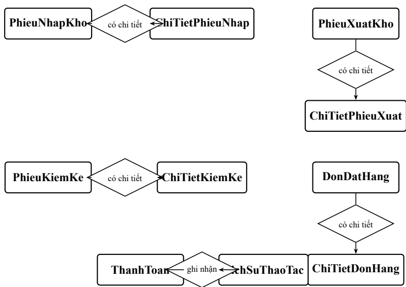
Hình 1: Sơ đồ ERD – Nghiệp vụ (Transaction)
